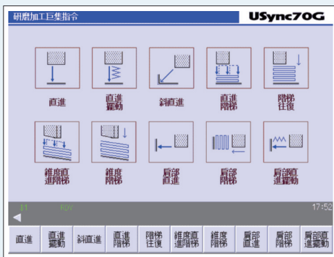
研磨循環總圖
